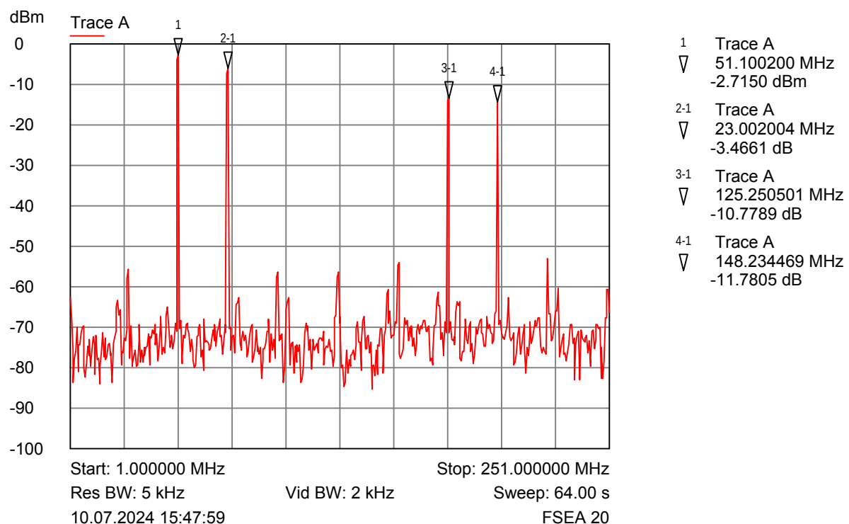
Bild 5 Tuning, Drive 100%, f=51MHz
