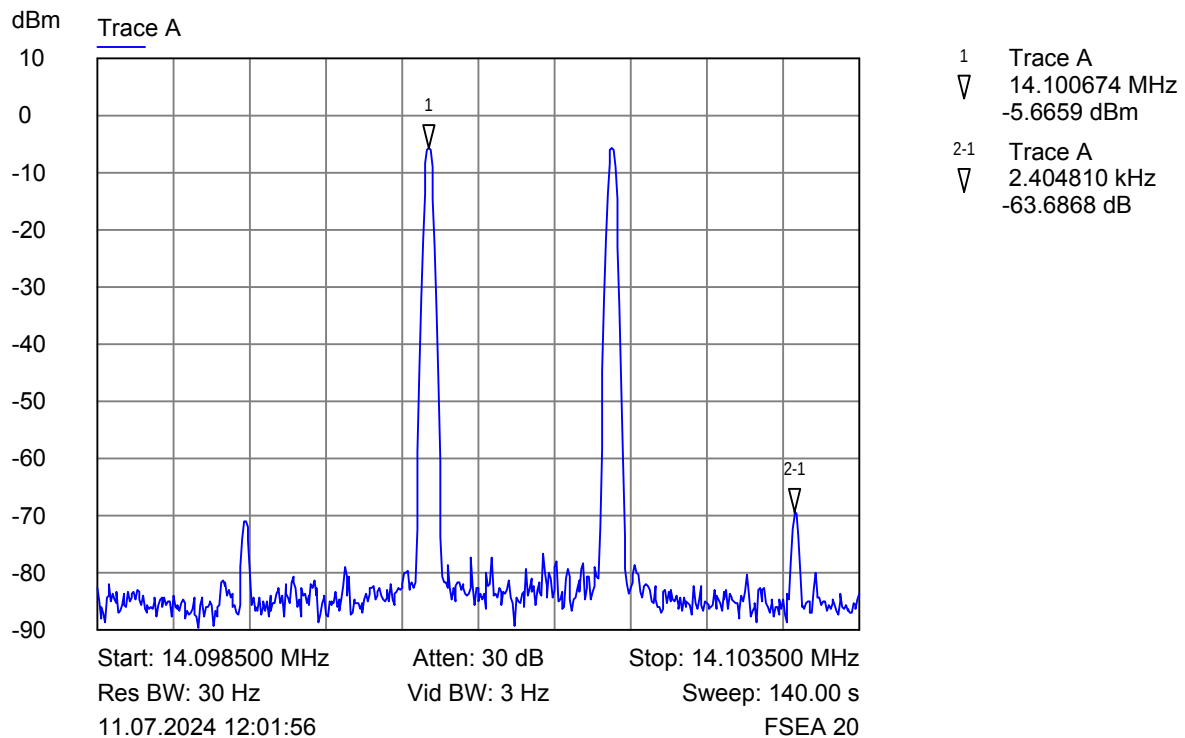
Bild 7 Produktbildung 3.Ordnung bei 14,1MHz und maximaler Leistung von 0dBm PEP
