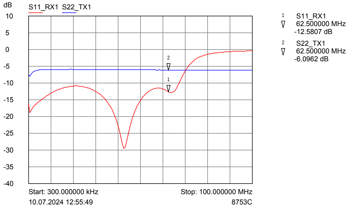
Bild 1 Reflexionsdämpfung am RX-Eingang und am TX-Ausgang
