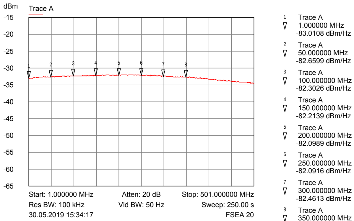
Bild 13 Messung an Ausgang 1. Ausgang 2 ist dabei abgeschlossen. Die Verstärkung ist über den Temperaturbereich wegen der internen Gegenkopplung der ICs sehr stabil. Bei einer Bandbreite von 500MHz beträgt die Summenleistung an jedem Ausgang -82 + 10 \cdot \log(500 \cdot 10^6) = +5\text{dBm} .
