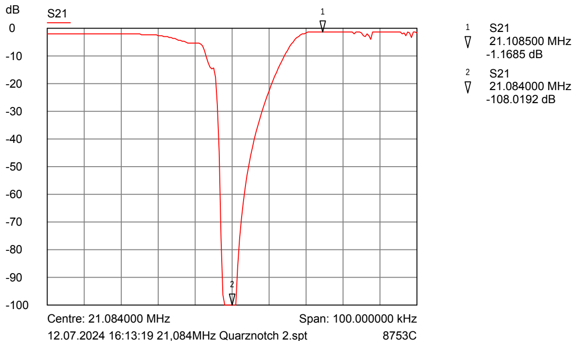
Bild 9 Das mit 7 Quarzen realisierte Notchfilter
