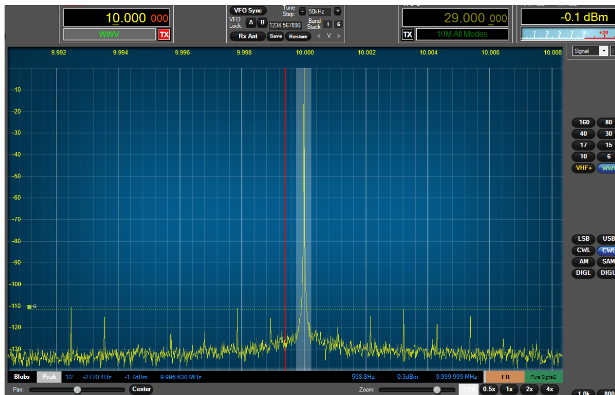
Bild 8 Hier sind die oben erwähnten Nebenwellen zu sehen.
