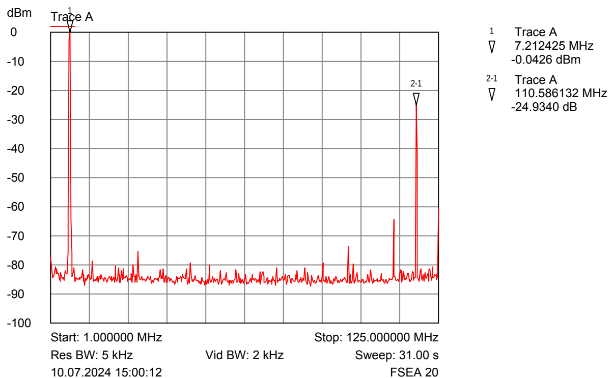
Bild 2 Tuning, Drive 100%, f=7,2MHz
