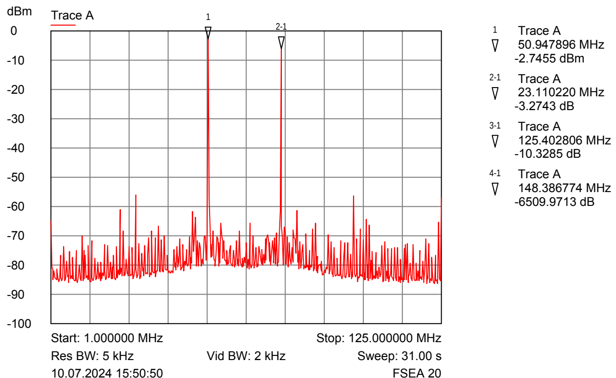
Bild 4 Tuning, Drive 100%, f=51\text{MHz}
