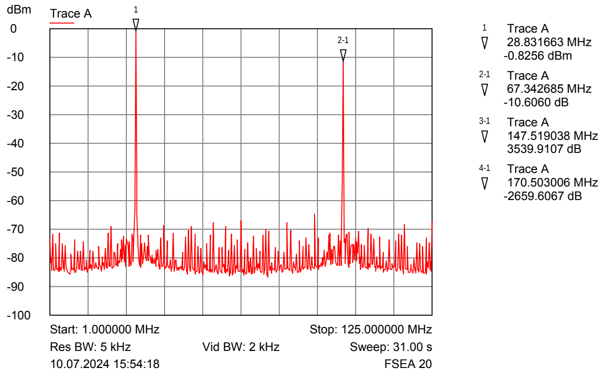
Bild 3 Tuning, Drive 100%, f=29\text{MHz}
