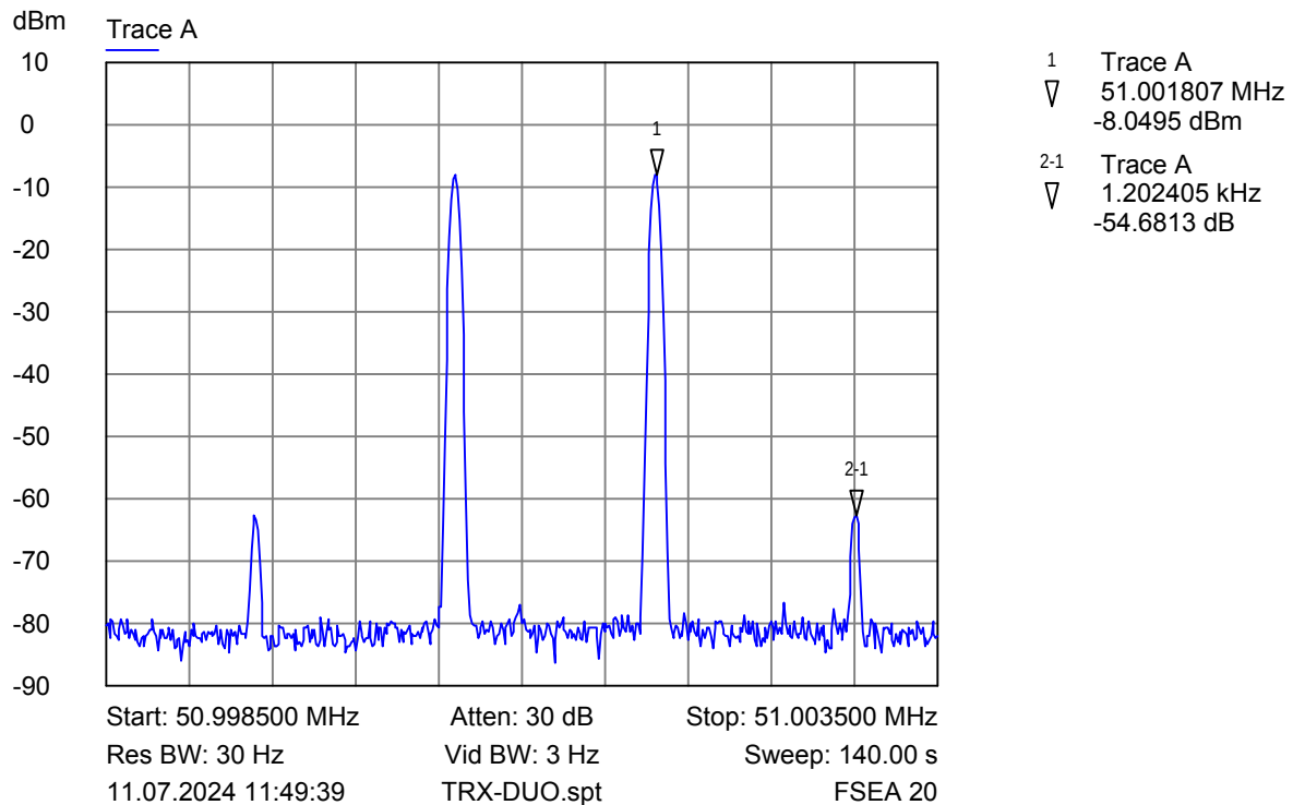
Bild 6 Produktbildung 3.Ordnung bei 51MHz und maximaler Leistung von -2dBm PEP
