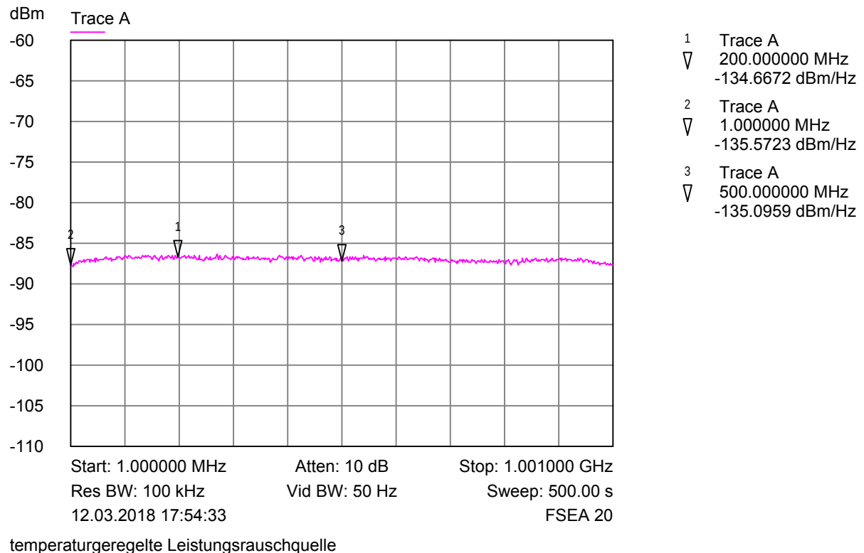
Bild 11 Die Rauschquelle gibt an einen 50Ω Widerstand -135dBm/Hz ab.
